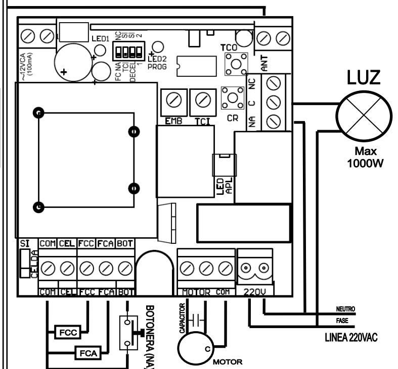
CONEXIÓN LUZ DE CORTESIA
