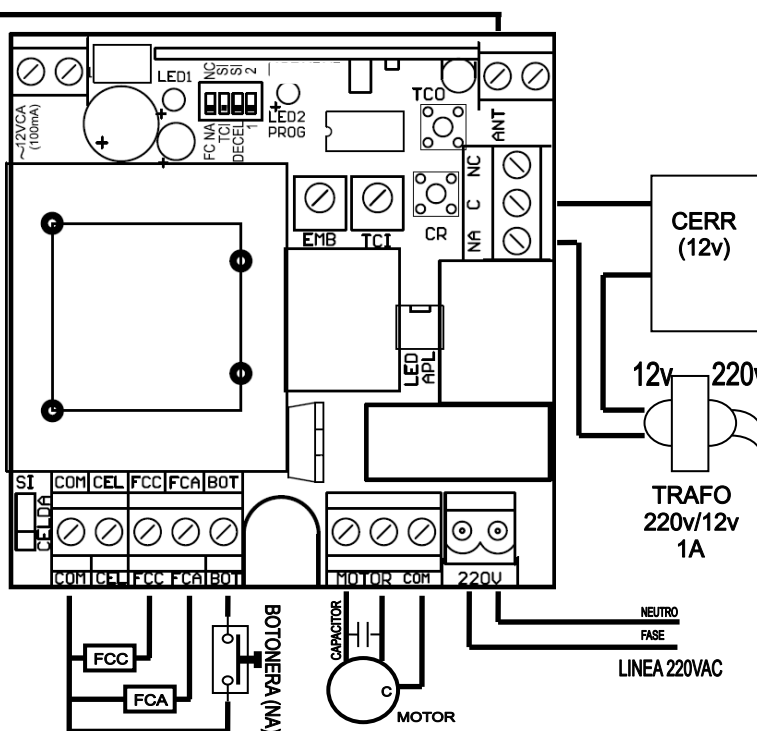
CONEXIÓN CERRADURA 12v
